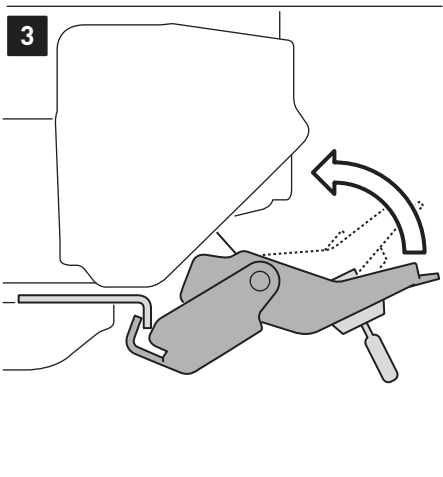
Spannverschluss Latch
